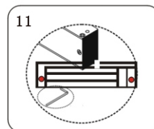
当确定所有安装步骤都正确无误, 吸力达到正常, 则最后步骤把防拆螺丝旋紧。
