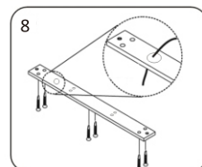
按已钻好的孔位旋紧螺丝固定吊装条
