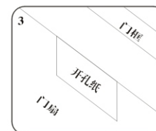
确定安装开孔纸位置后, 依照开孔纸上标示吸板与磁力锁的孔位。
