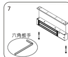
先将锁体吊装条拆除
