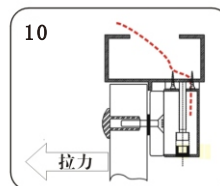
关门并测试吸力, 可增减垫片或转紧吸板来调整吸板和磁力锁吸附面的间隙
