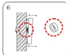
橡胶垫片的作用在于使吸板能微微调动, 让吸板和磁力锁吸附面能紧密贴合面无间隙, 吸力达到最高。
