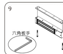
用六角板手把内六角螺丝固定磁力锁体于吊装条上。
