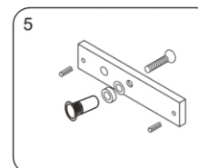
依照图示组合吸板 (不同的门板所钻的孔孔径有所不同, 请参照附图)
