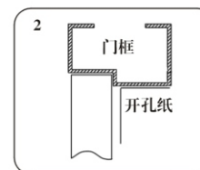
关上门后, 安装开孔纸置于靠近门框顶端以及门轴另一端位置。
