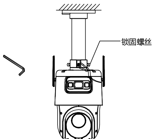
图2-13 固定设备
