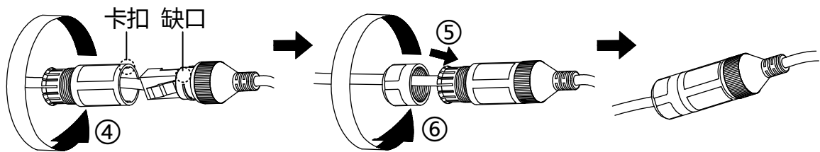
图2-16 完成安装
