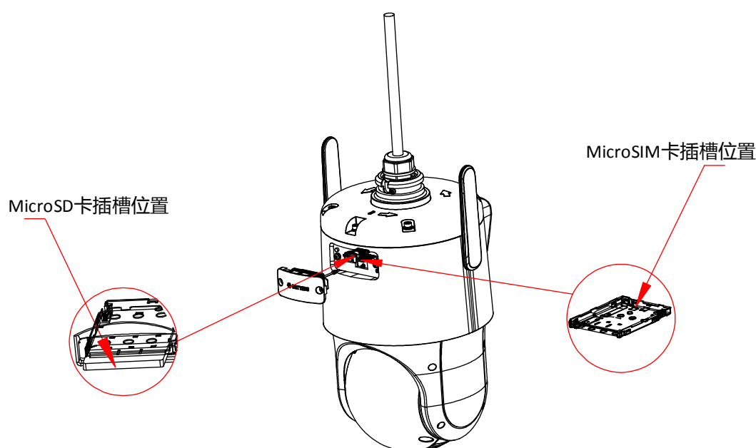
图2-3 MicroSIM 卡和 MicroSD 卡插槽位置
