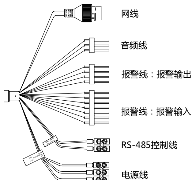
图2-2 一体化辫子线
