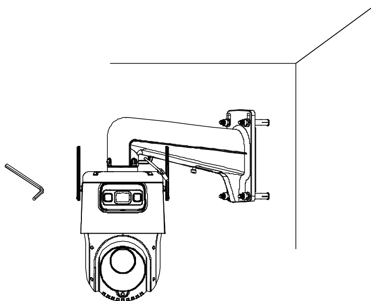
图2-6 固定设备
