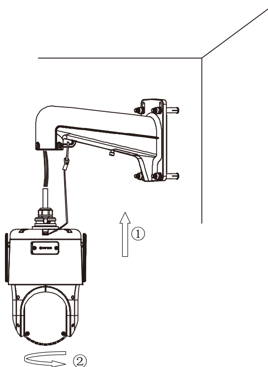
图2-5 拧入设备
