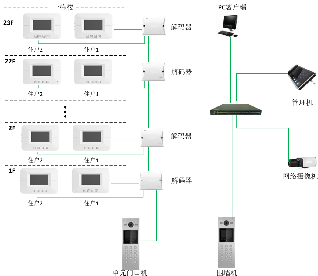
图1-1 系统架构示意图
